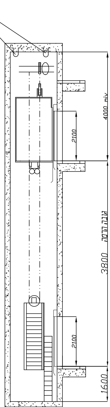
חתך 1-1 תכנית הרכבה
