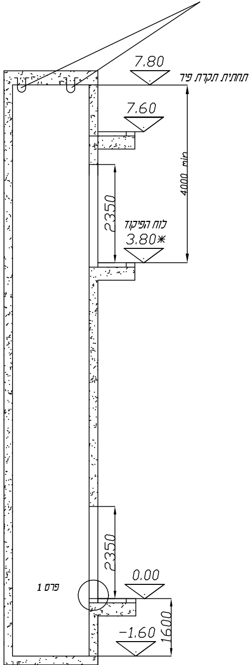
חתך 1-1 תכנית בניה
