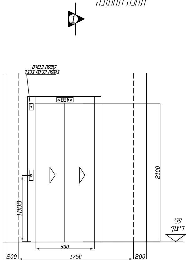
מבט חזית - תחנה תחתונה
