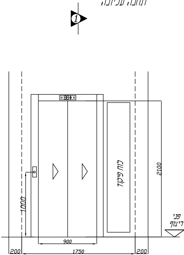
מבט חזית - תחנה עליונה
