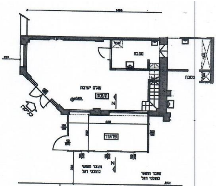
חכנית פרגוד ק.מ.100
