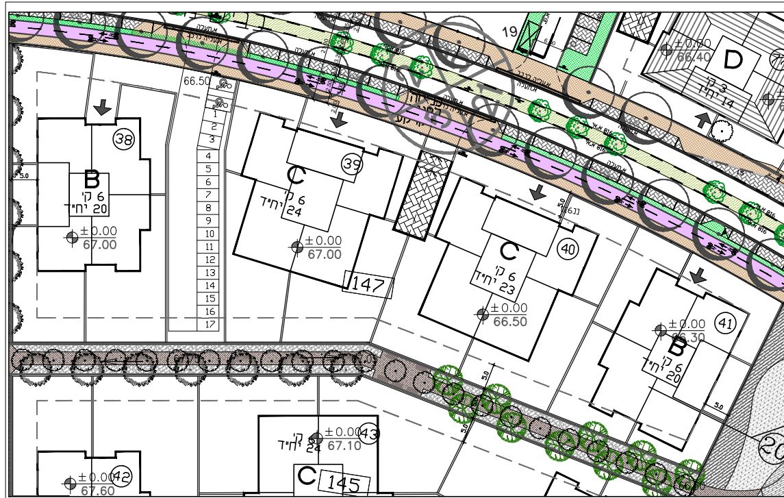
תכנית מגרש מס' 147 ק.מ. 1:1000
