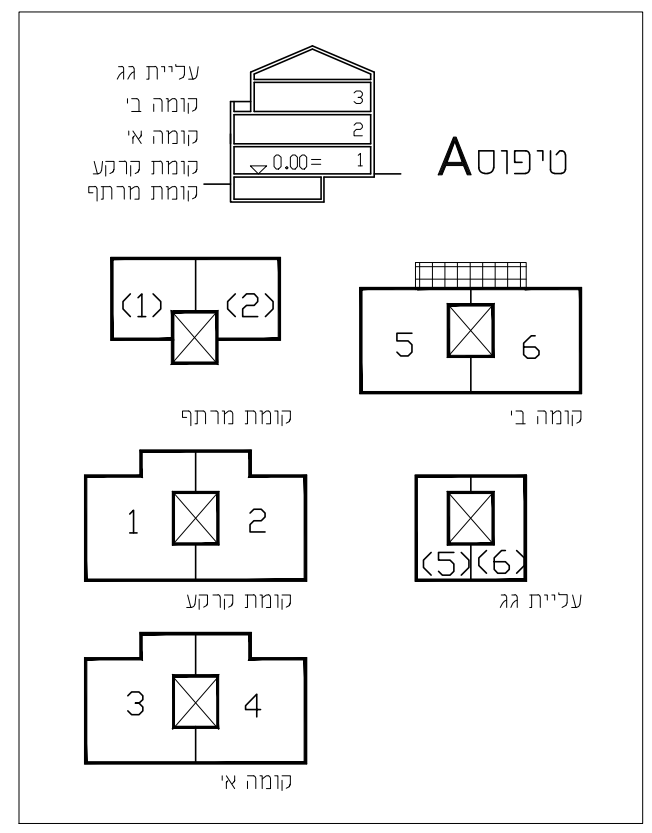
סכמת התפלגות יחיד בבנינים מס' 52,51,50,49
