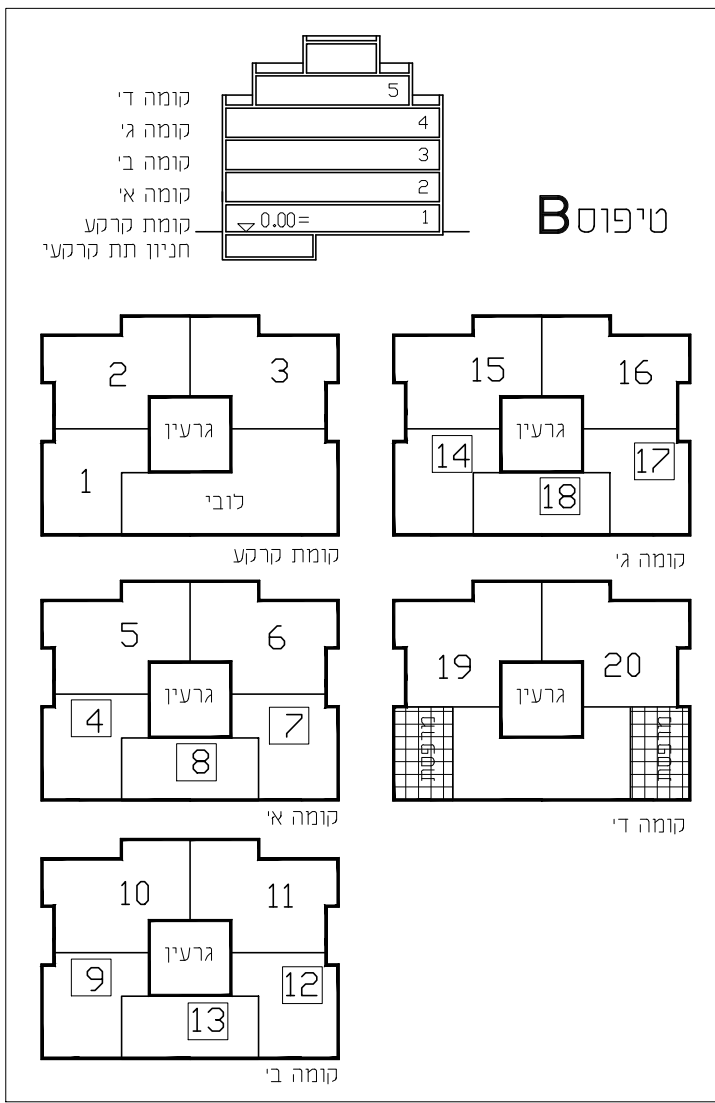
סכמת התפלגות יחיד בבנינים מס' 47,46,45 יחיד קטנות ב 3 בנינים
