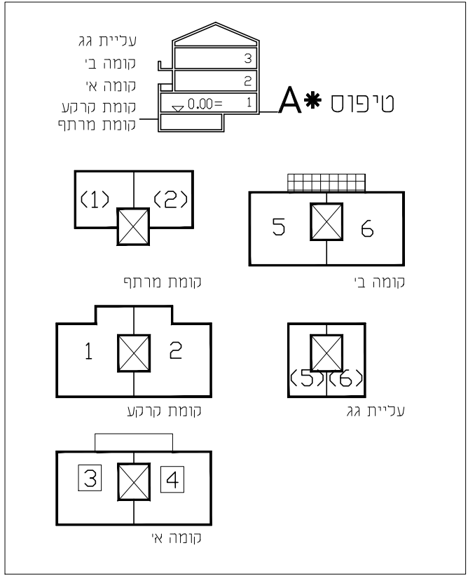
סכמת התפלגות יחיד בניין מס' 73,74 יחיד קטנות ב-2 בנינים 4
