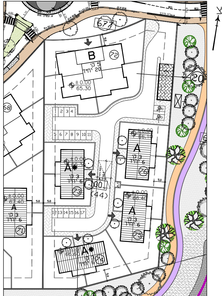
תכנית מגרש מס' 100 ק.מ. 1:1000
