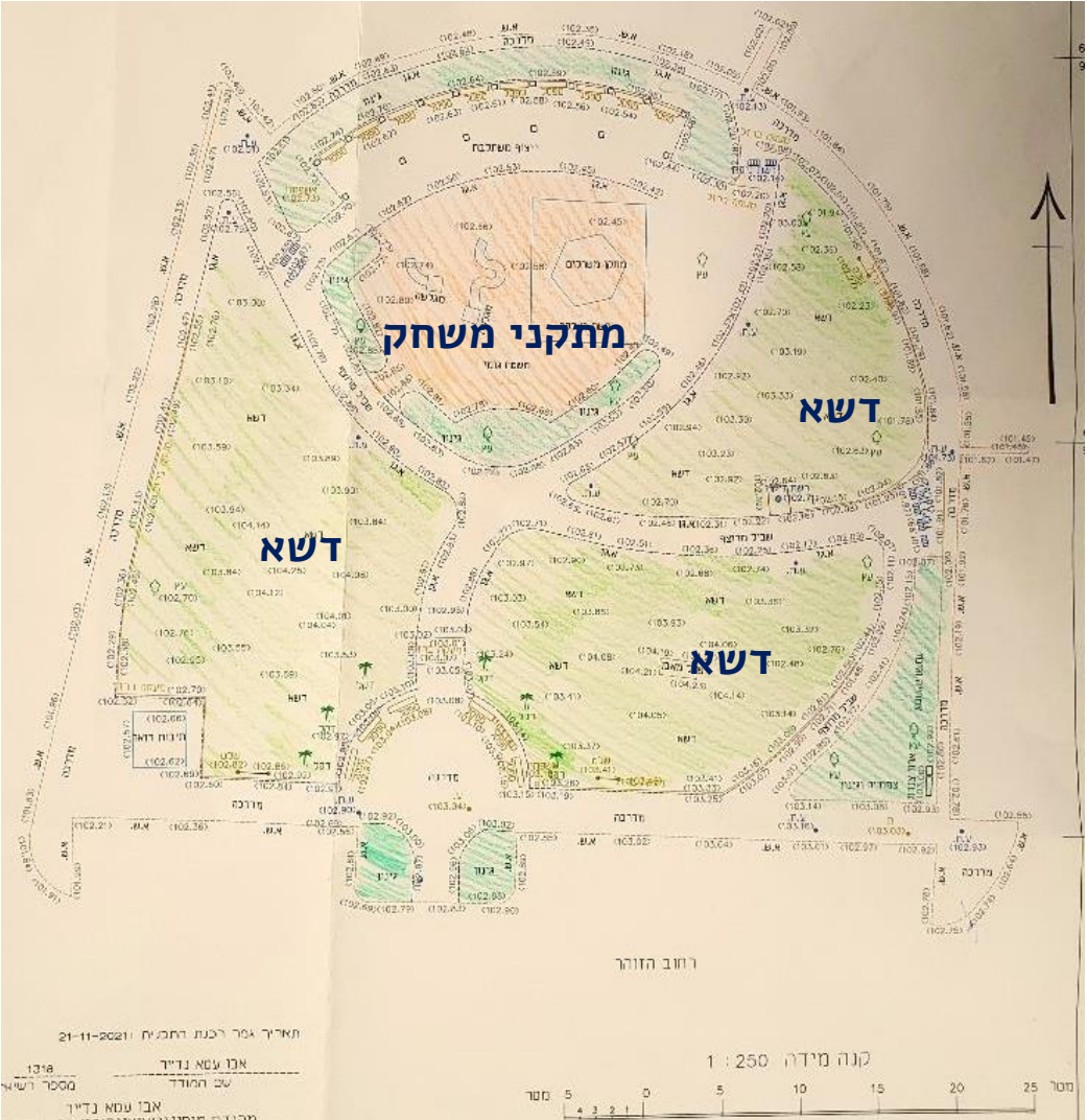
תכנית מדידה
