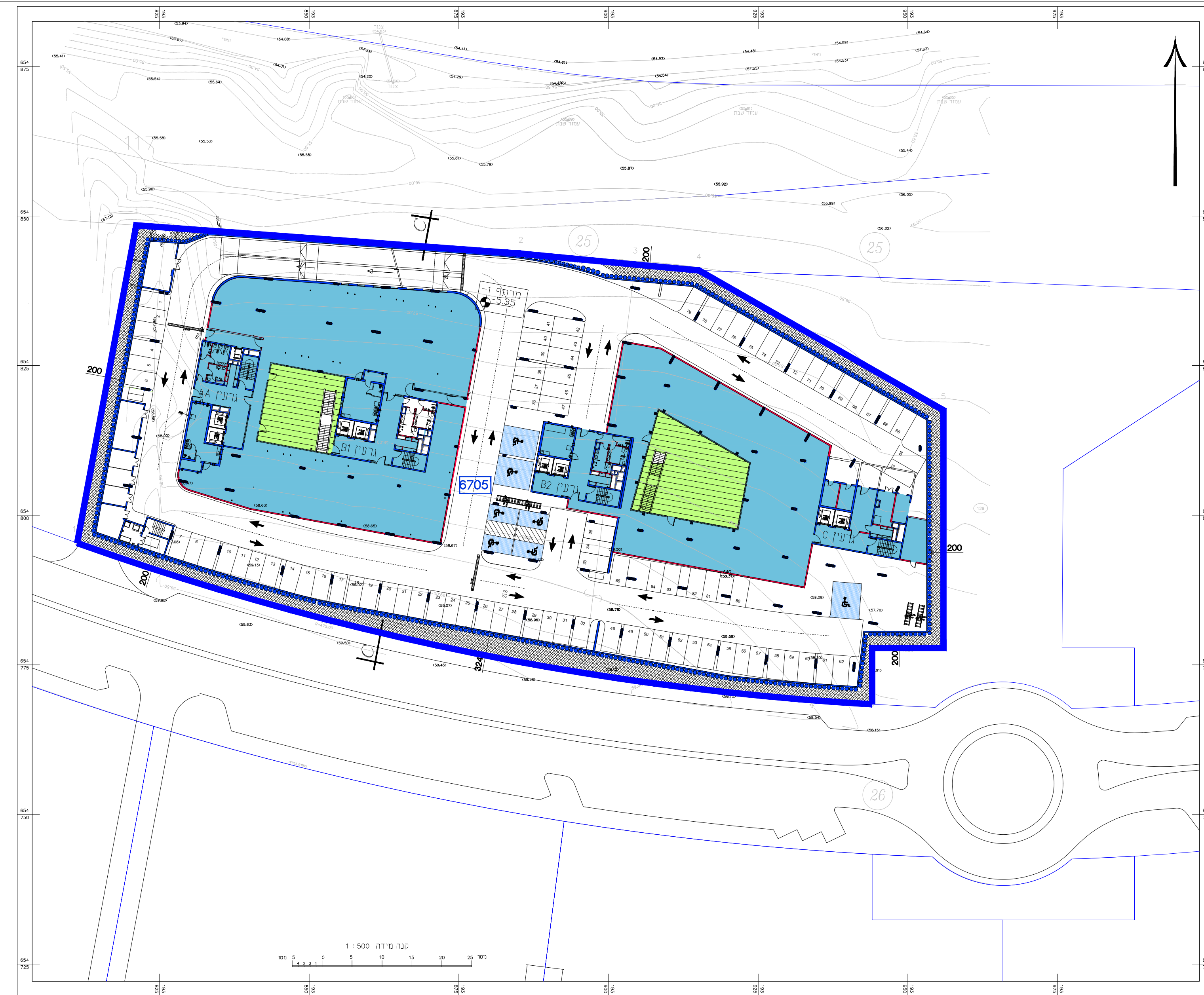
תכנית קומת מרתף 1- קנ"מ: 1:500
