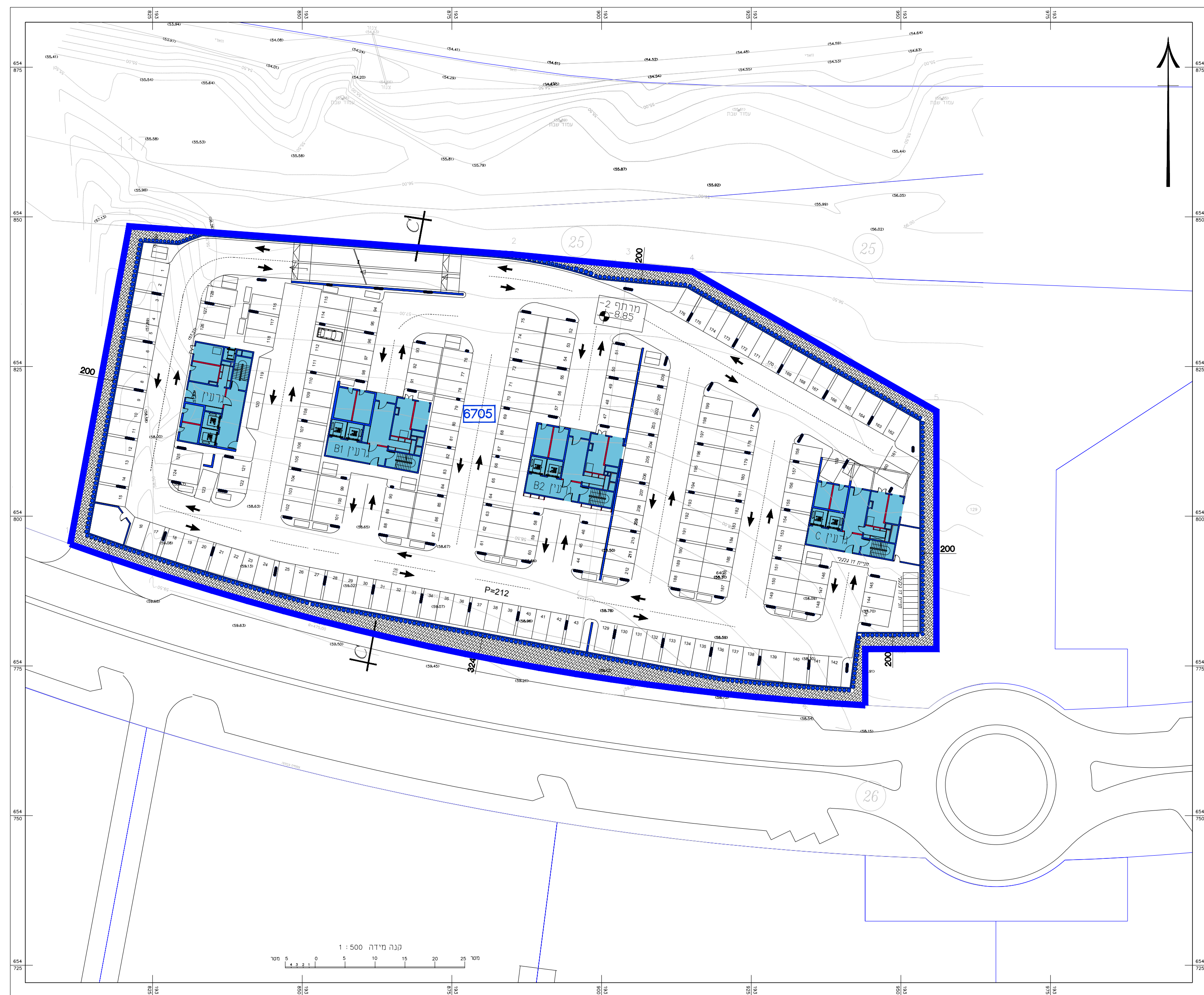
תכנית קומת מרתף 2- קנ"מ: 1:500
