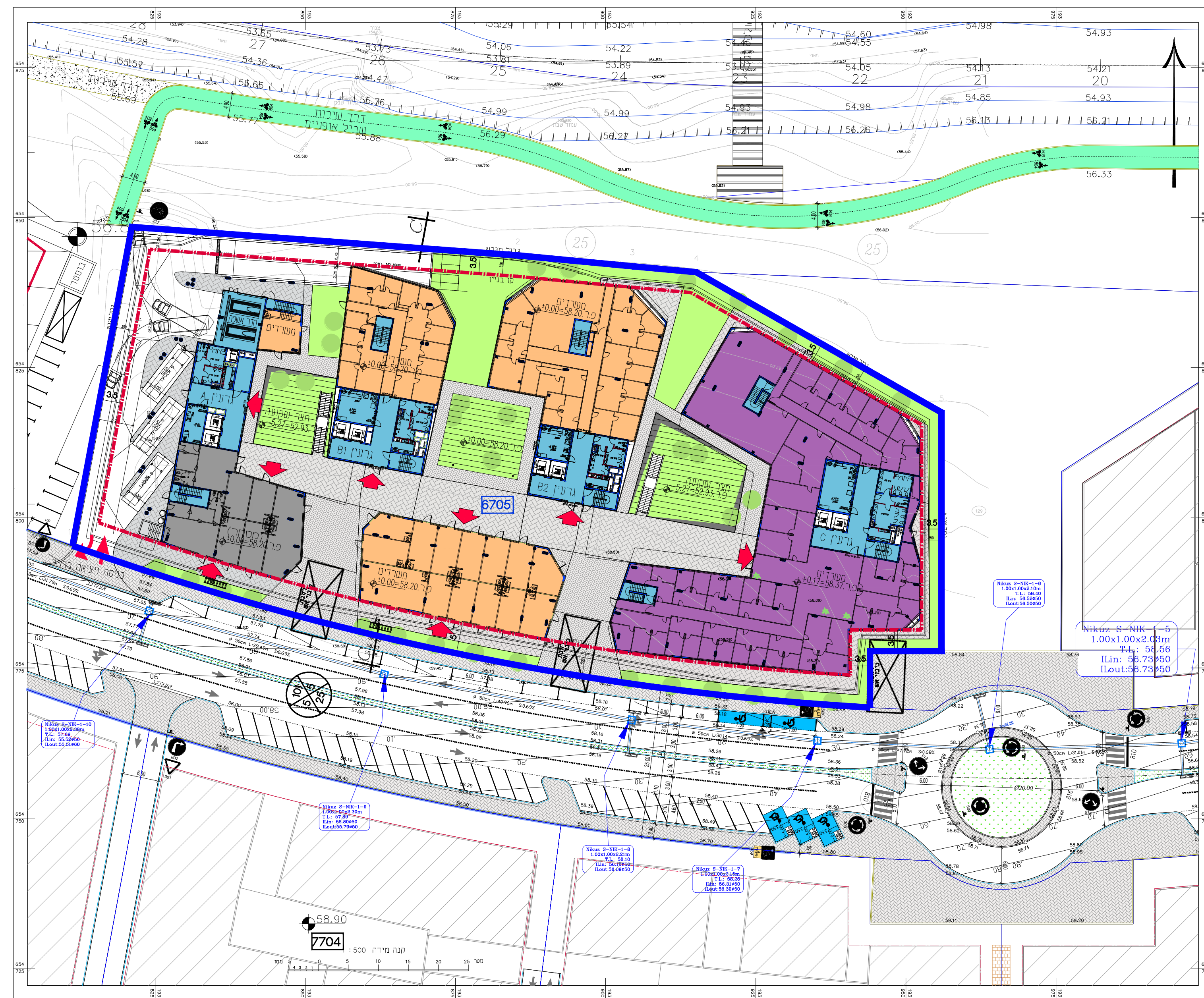
תכנית קומת קרקע קנ"מ: 1:500
