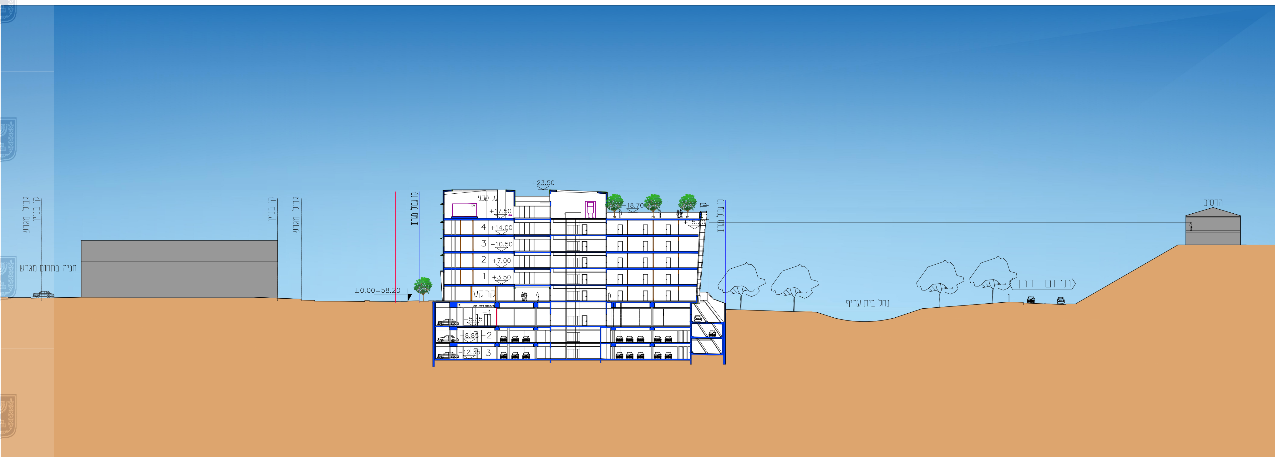
חתך C-C קנ"מ: 1:500
