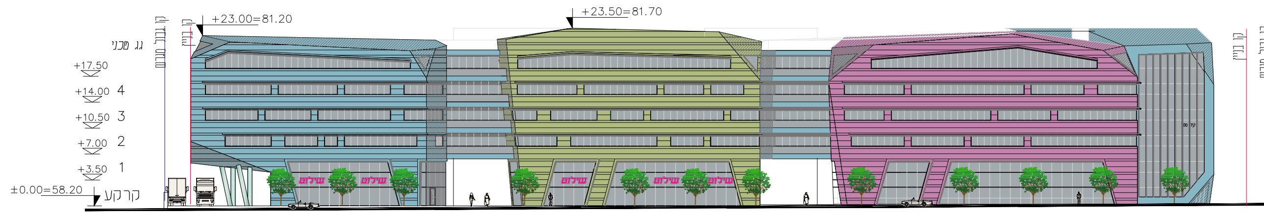
חזית דרומית קנ"מ: 1:500
